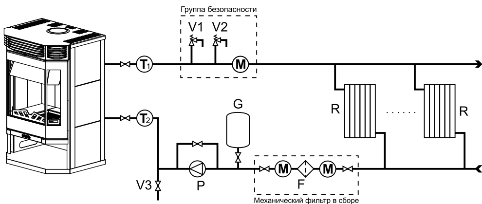
Рис.3.3. Схема подключения печи-камина “Аква” к системе отопления
