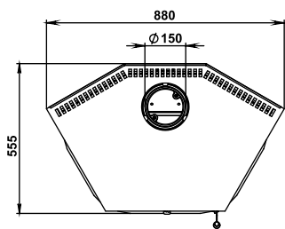
Рис.2.9. Печь-камин "Москва 12" (АОТ-12-01)
